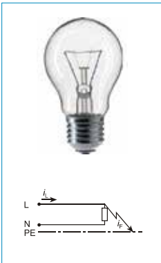
Typ AC
